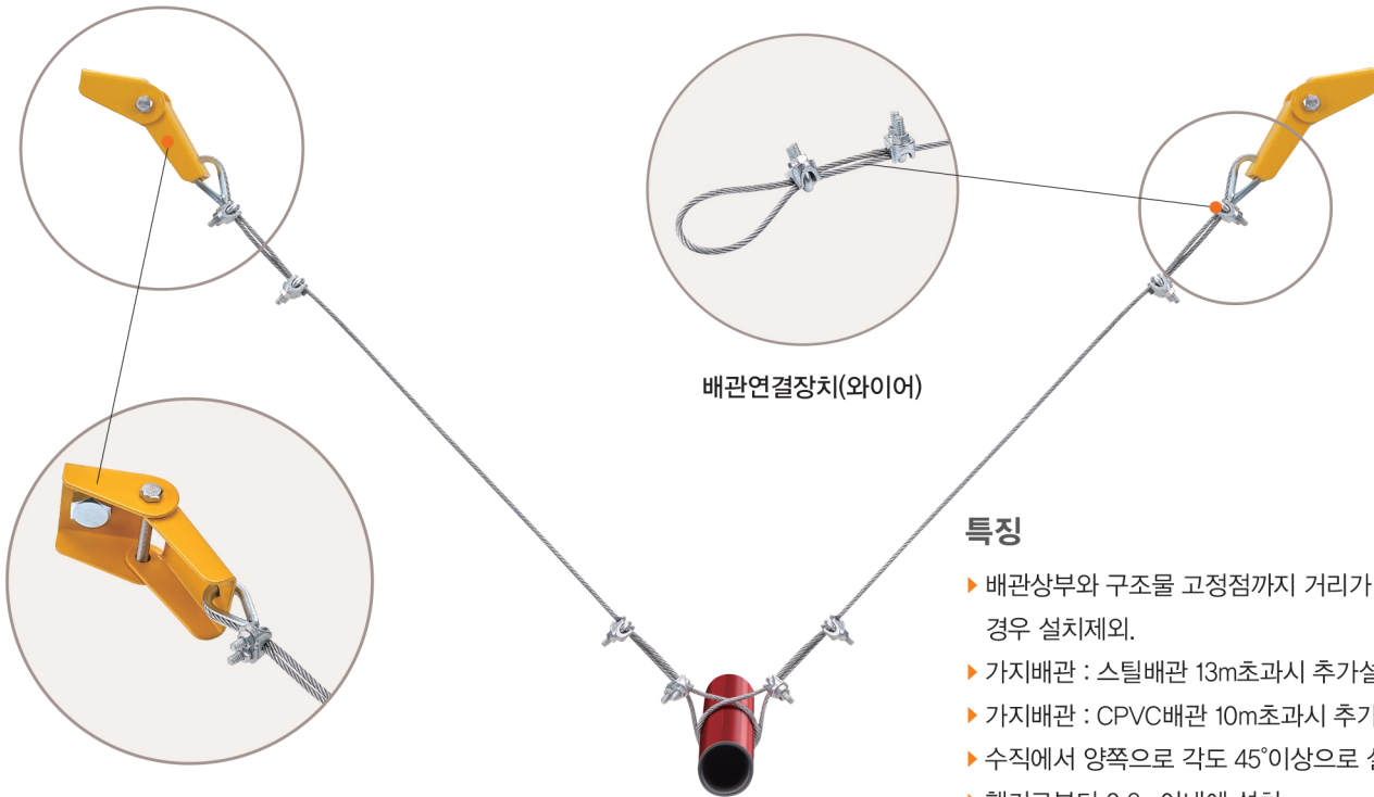
건축물부착장치
